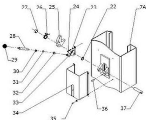
Dispositivo de proteção do lado da energia
