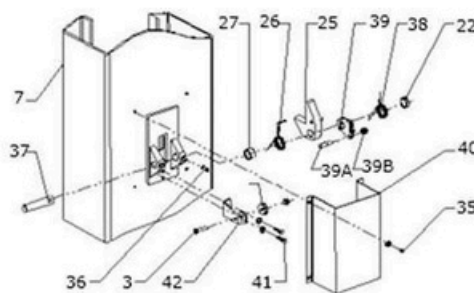
Dispositivo de proteção do lado sem energia
